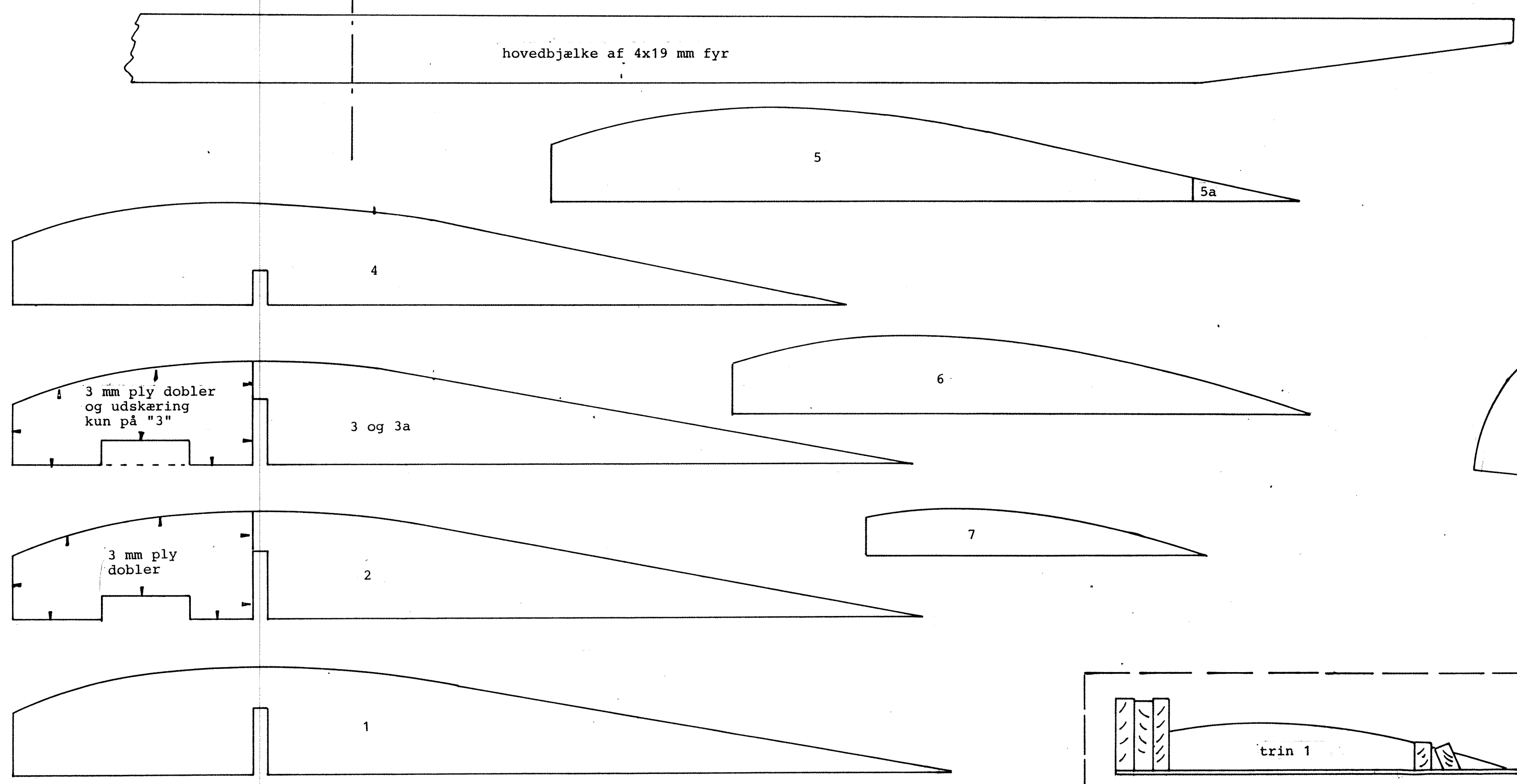
ALLE RIBBER AF 3 MM BALSA
